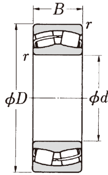
円筒穴
